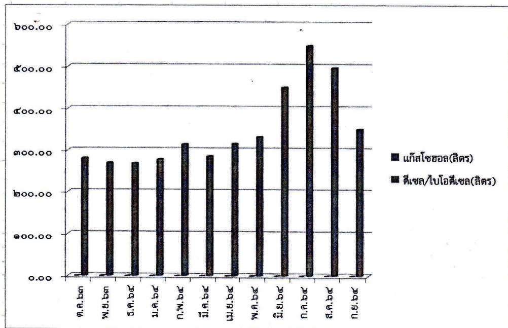
แผนภูมิ ๒ สถิติปริมาณการใช้เชื้อเพลิง ประจำเดือนตุลาคม ๒๕๖๓ – เดือนกันยายน ๒๕๖๔
